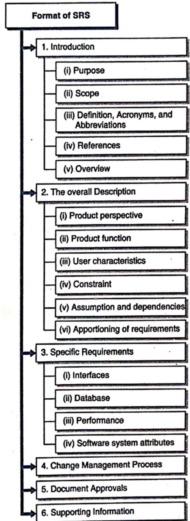
Fig. 2.5.2 : Format of SRS
